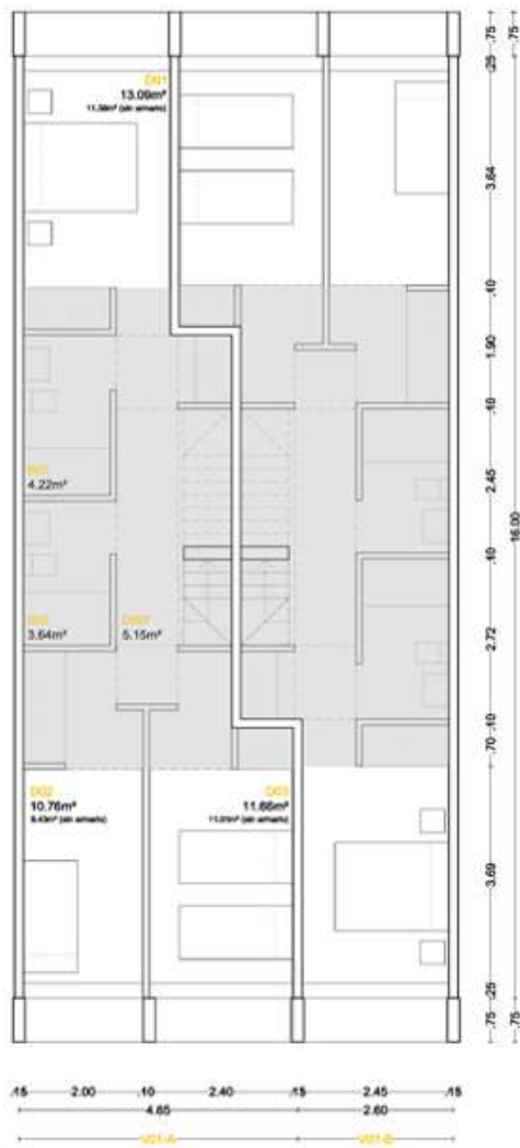
PLANTA PRIMERA
