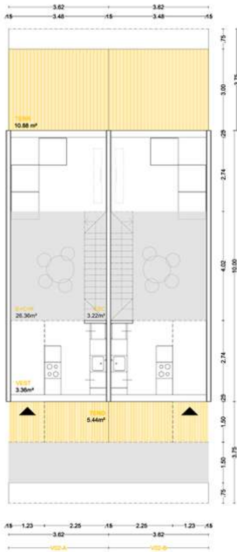
PLANTA ÁTICO
